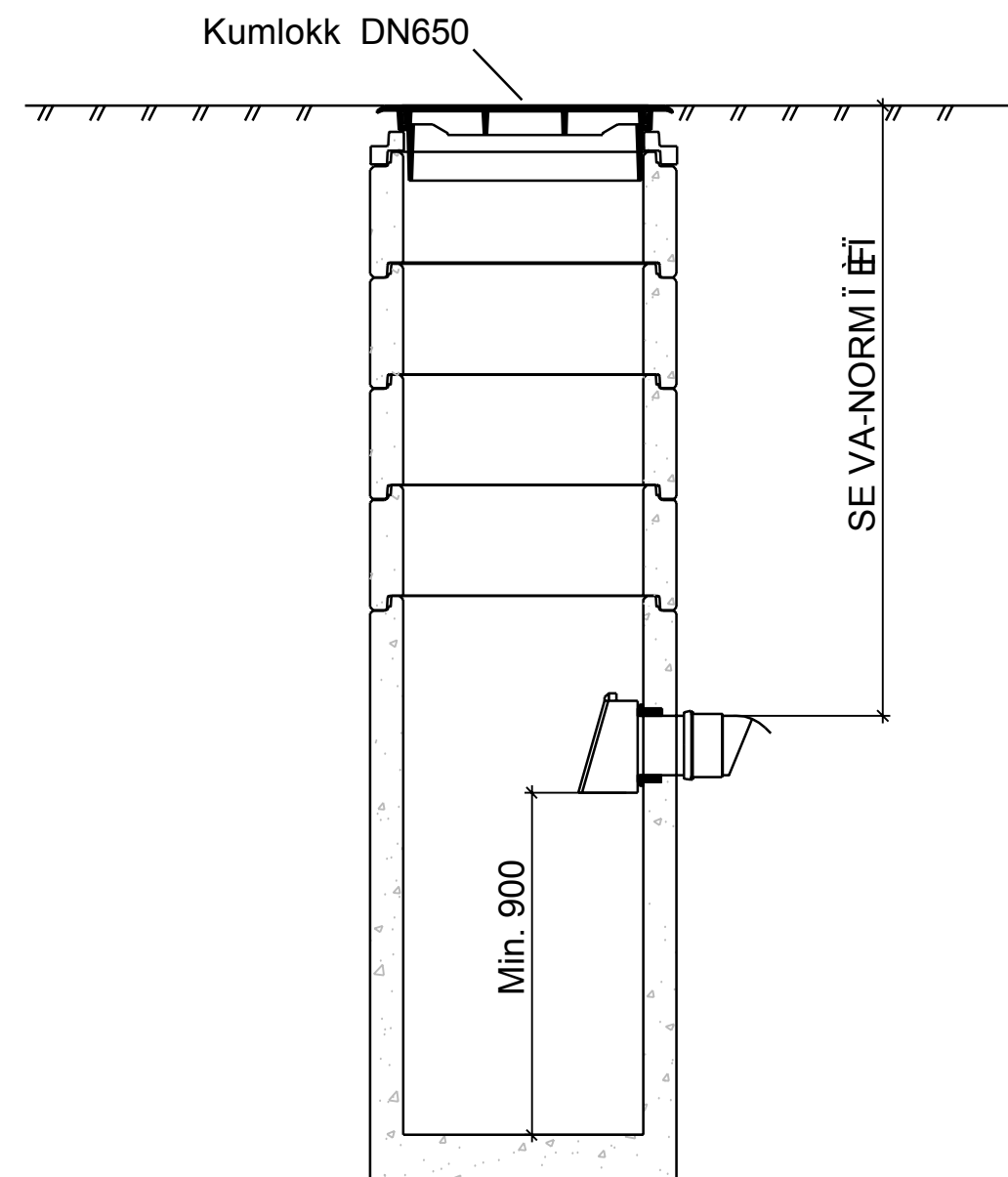
SNITT SANDFANGSKUM BETONG 650 MM - 120 -
