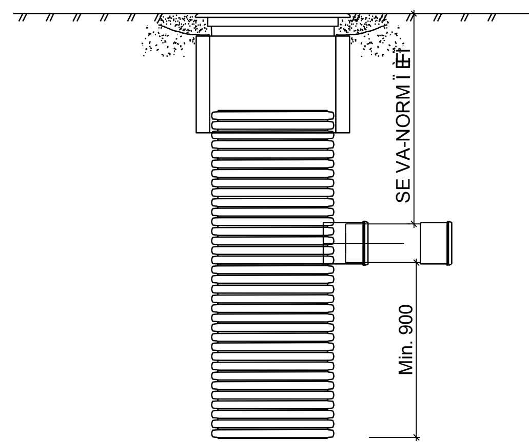
SNITT SANDFANGSKUM 630 MM - 120 -
