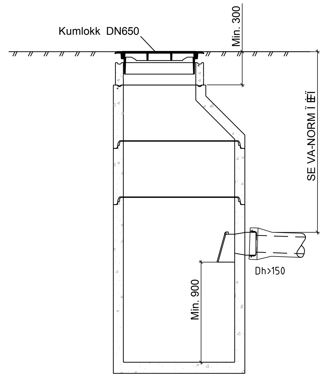
SNITT SANDFANGSKUM BETONG 1000 MM - 120 -
